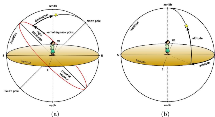
Figura 1: I sistemi di coordinate equatoriali e altazimuthali.
